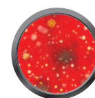
citi alerģēni
