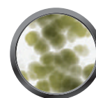
pelējuma sporas
