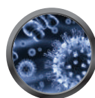
vīrusi
